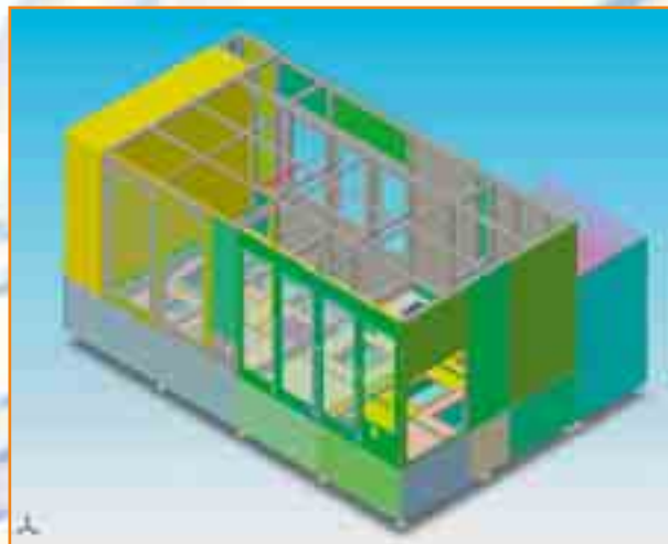
Kompletthanlage mit Verkleidung, Schiebetüren, Tank-einheiten und Anbauteilen; Gestelllänge 5400 mm
